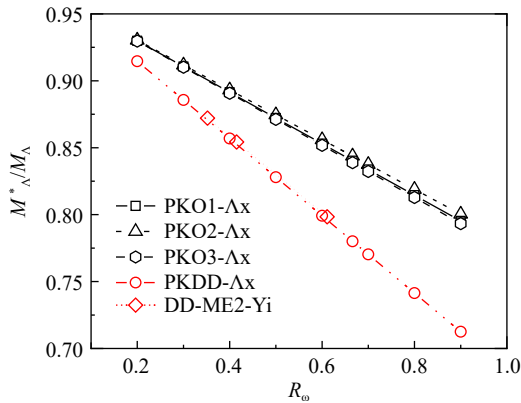
图 3 含超子核物质中超子 M_{\Lambda}^*/M_{\Lambda} 随矢量耦合强度比值 R_{\omega} 的变化(在线彩图)
