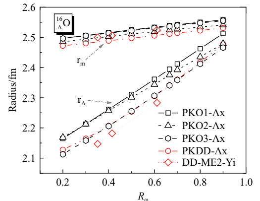
图 4 采用 RHF 有效相互作用 PKO1- \Lambda x, PKO2- \Lambda x, PKO3- \Lambda x(黑色)以及 RMF 有效相互作用 PKDD- \Lambda x, DD-ME2-Yi(红色)计算给出的 ^{16}_{\Lambda}\text{O} 超核物质半径及 \Lambda 超子半径随矢量耦合强度比值 R_{\omega} 的变化(在线彩图)
