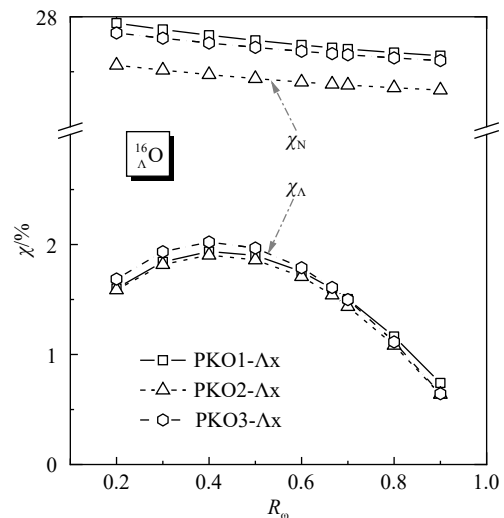
图 2 采用 RHF 有效相互作用 PKO1- \Lambda x、PKO2- \Lambda x 和 PKO3- \Lambda x 计算的 {}^{16}_\Lambda\text{O} 超核中核子与超子道交换项与直接项能量泛函比值 \chi 随 R_\omega 的变化
