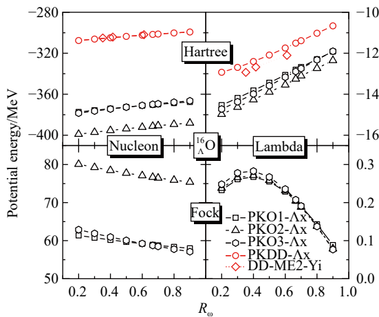
图 1 采用不同 CDF 有效相互作用给出的核子、超子的直接项与交换项势能随耦合强度比值 R_\omega 的变化
